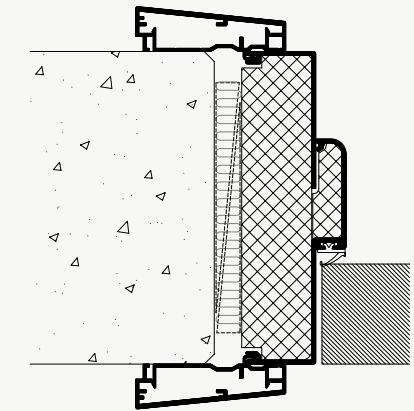
DEKO TD - TRÆDØR ALUMINIUMINDFATNING TYPE ASIF
