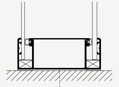
GULVTILSLUTNING
