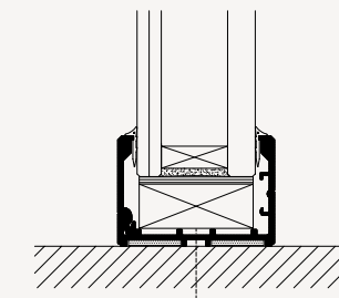
GULVTILSLUTNING
