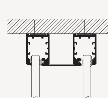
LOFTTILSLUTNING
