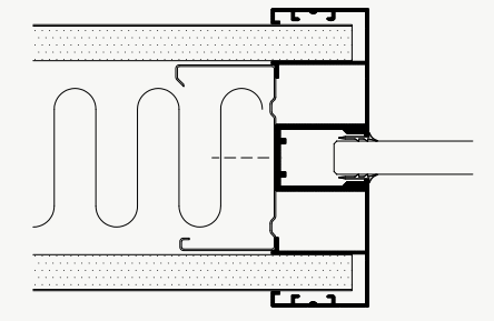
GIPS-/DEKO FG-SAMLING
