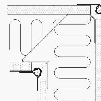
HJØRNE
