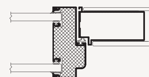
DEKO DG - GLASDØR
