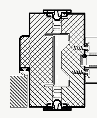
DEKO TD - TRÆDØR
