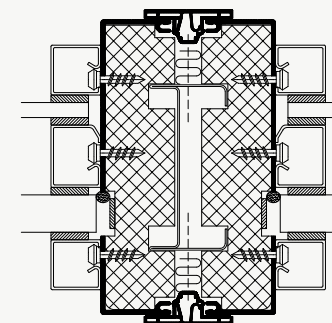
GLASSAMLING 2 LAG GLAS
