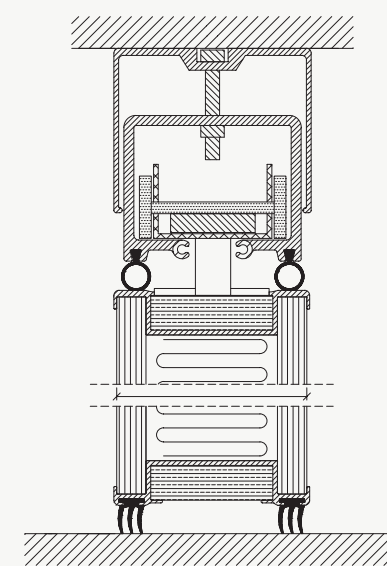
TOPHÆNGT LOFT- OG GULVTILSLUTNING
