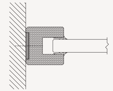
VÆGTILSLUTNING
