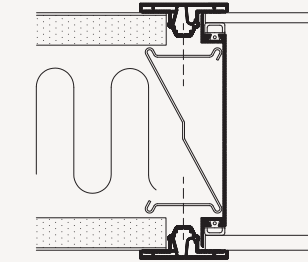
GLAS-/GIPSSAMLING
