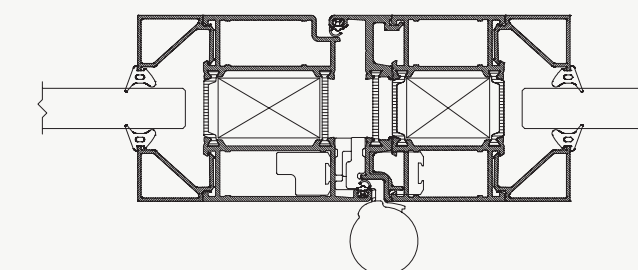
DEKO AG - ALUMINIUMGLASRAMMEDØR
