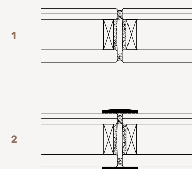
GLASSAMLING
