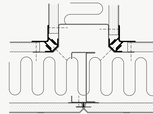
TVÆRVÆGSSAMLING
