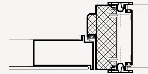
DEKO DG - GLASDØR
