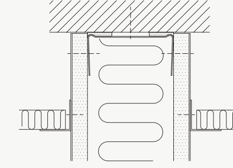
LOFTTILSLUTNING
