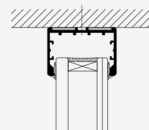
LOFTTILSLUTNING
