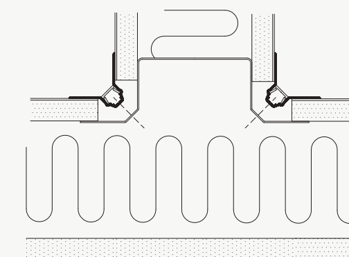
TVÆRVÆGSSAMLING
