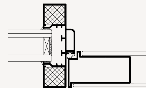
DEKO DG - GLASDØR
