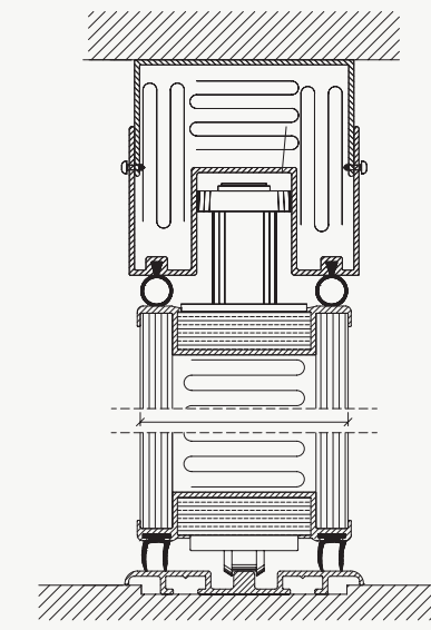
GULVKØRENDE LOFT- OG GULVTILSLUTNING
