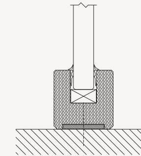
GULVTILSLUTNING
