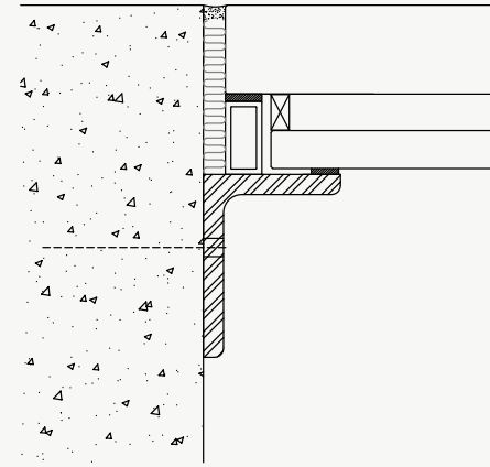
KANTUNDERSTØTNING
