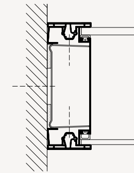
VÆGTILSLUTNING
