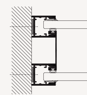
VÆGTILSLUTNING
