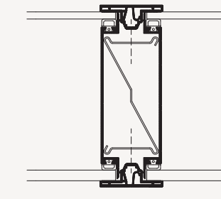
GLASSAMLING
