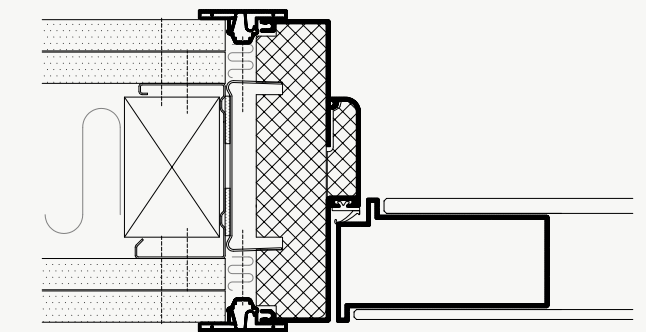
DEKO DG - GLASDØR ALUMINIUMINDFATNING TYPE ASPD
