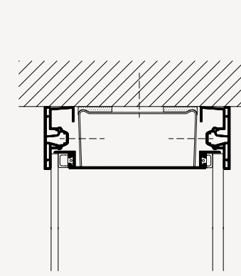
LOFTTILSLUTNING
