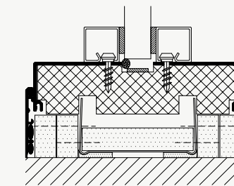
GULVTILSLUTNING
