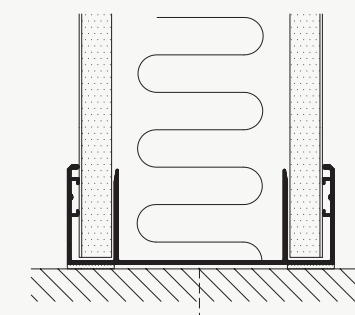
GULVTILSLUTNING
