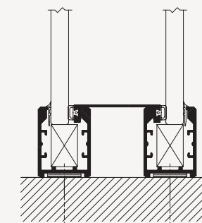
GULVTILSLUTNING
