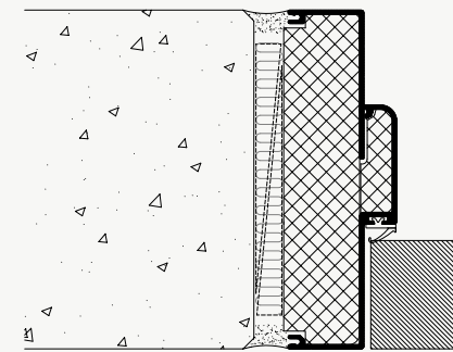
DEKO TD - TRÆDØR FUGET OVERGANG
