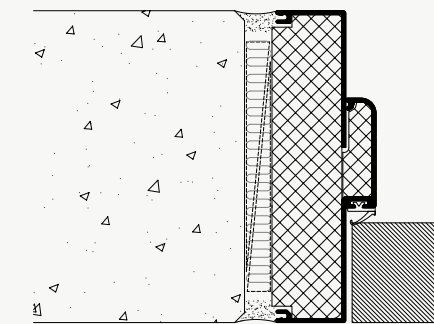
DEKO TD - TRÆDØR FUGET OVERGANG
