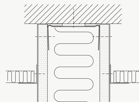
LOFTTILSLUTNING
