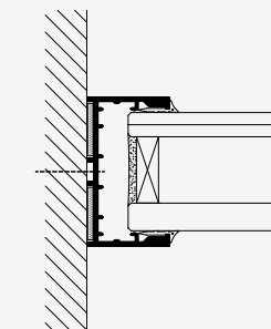
VÆGTILSLUTNING
