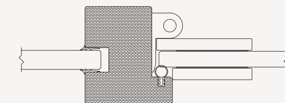
DEKO FD - FULDGLASDØR
