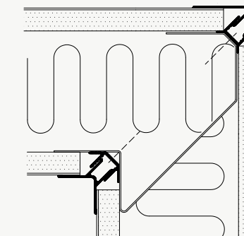
HJØRNE
