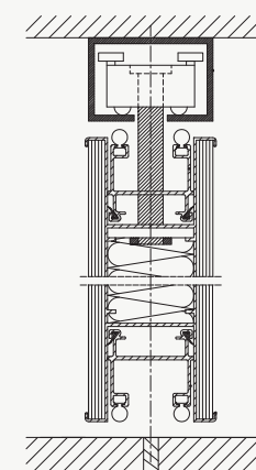
GULV- OG LOFTTILSLUTNING
