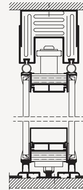
GULV- OG LOFTTILSLUTNING
