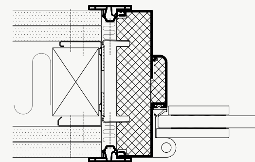
DEKO FD - HELGLASDØR ALUMINIUMINDFATNING TYPE ASPD
