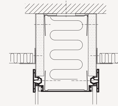
LOFTTILSLUTNING
