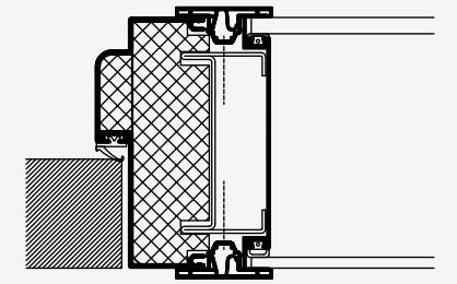
DEKO TD - TRÆDØR
