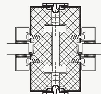
GLASSAMLING 1 LAG GLAS
