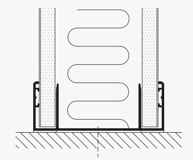
GULVTILSLUTNING
