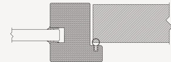
DEKO TD - TRÆDØR
