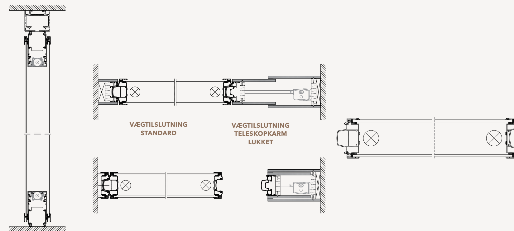
LOFT- OG GULVTILSLUTNING
