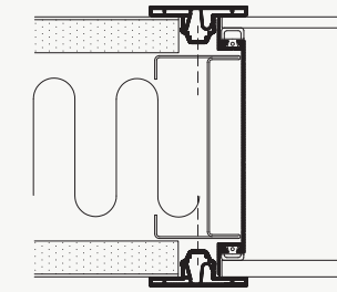
GIPS-/GLASSAMLING
