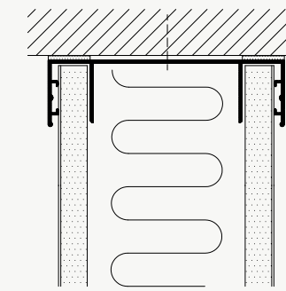
LOFTTILSLUTNING
