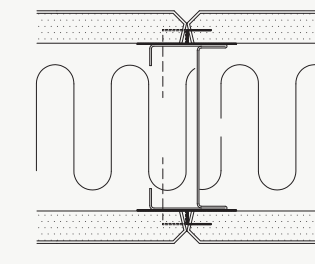
GIPS-/GIPSSAMLING
