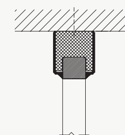
LOFTTILSLUTNING
