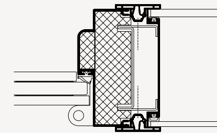
DEKO FD - FULDGLASDØR
