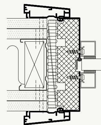
VÆG-/GLASSAMLING
