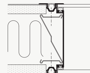
GIPS-/GLASSAMLING
