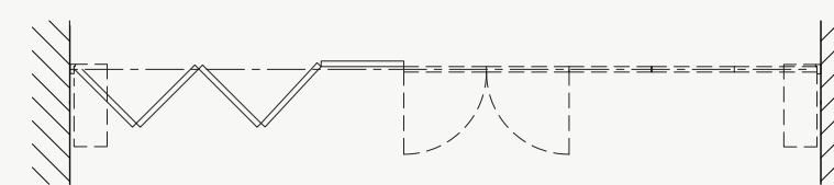
SIDEHÆNGT DOBBELTFLØJET
