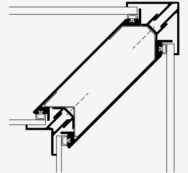
HJØRNESAMLING
