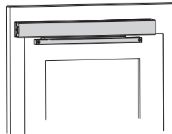
Hovedmontage med glideskinne
