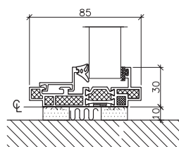
Profil ved gulv
