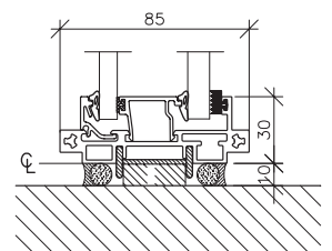
Profil ved gulv.
