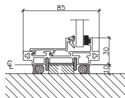
Profil ved gulv.
