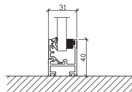
Profil ved gulv
