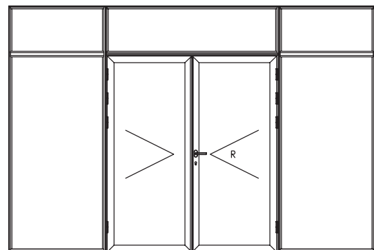
ID85 dobbeltglas parti med dobbeltdør.
