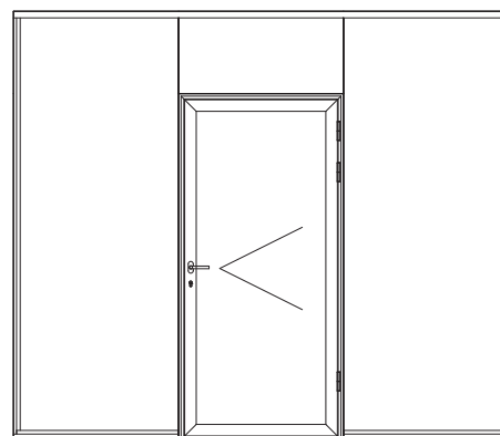
ID31 parti med glasrammedør og overparti
