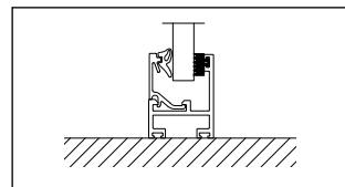
ID31 helglas.
