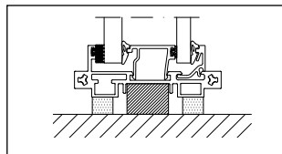
ID85 dobbeltglas.
